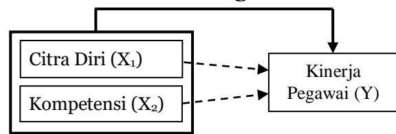
Gambar 1. Kerangka Pemikiran
